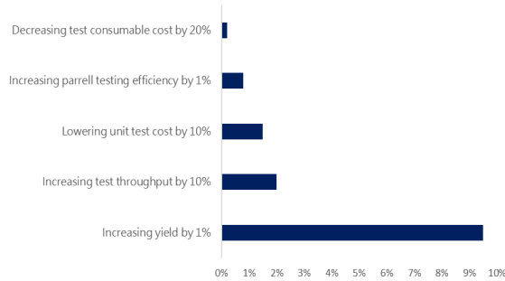
圖 4：提升晶片良最終率對成本下降效益最大
