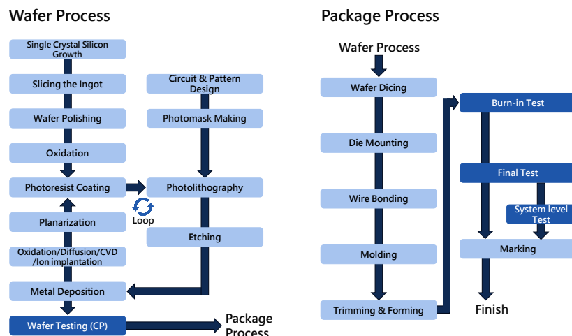
圖 6：半導體測試流程主要分為前端 (CP) 和後端 (FT)
